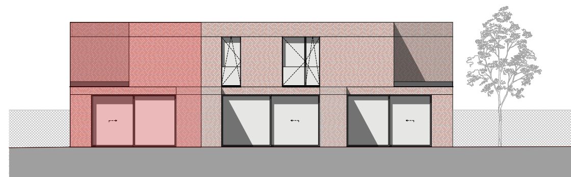
ACHTERGEVEL
